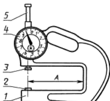
1 — корпус; 2 — пятка; 3 — измерительный наконечник; 4 — отсчетное устройство; 5 — измерительный стержень; A — вылет
